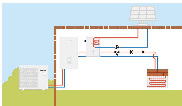
Aquarea J- und H-Generation: Heizungssystem mit Aquarea Splitsystem, Pufferspeicher, Solarthermianlage und Mischventil
